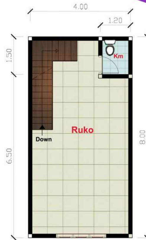
DENAH LT.DUA
